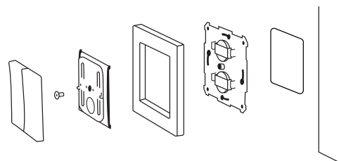
Montage med medföljande tejp på vägg/kakel.
