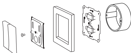
Montage utanpå apparatdosor med skruv.
