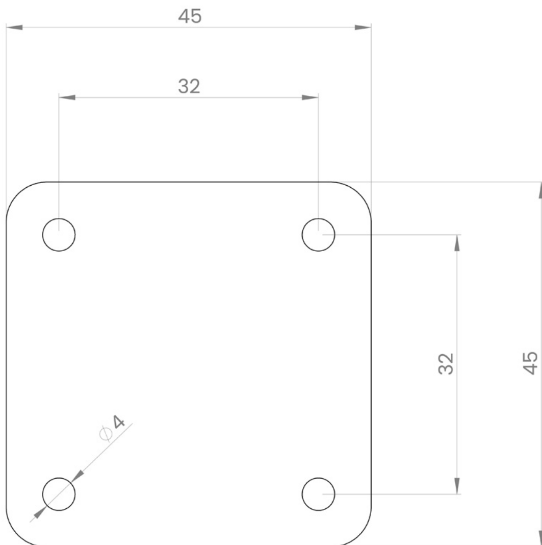
Kiinnitysreikien mitoitus - mounting hole spacing
