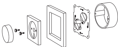
Montage utanpå apparatdosa med skruv.
