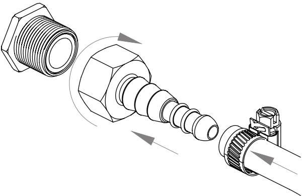
Flaschenventilgewinde
