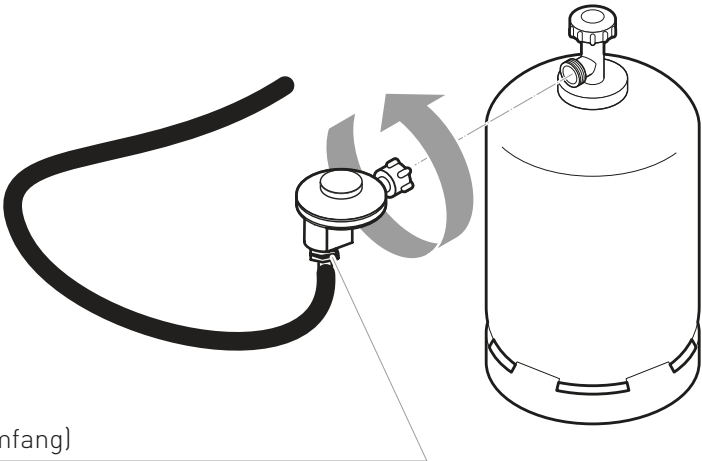
Flaschenventilgewinde
