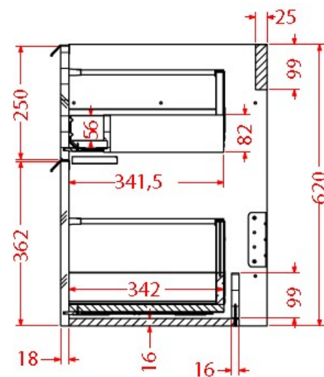
SEZIONE A-A
