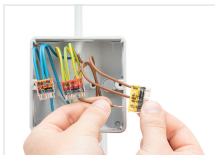
Anslutning: Anslut den skalade ledaren tills den tar emot bakkanten inuti klämmen
