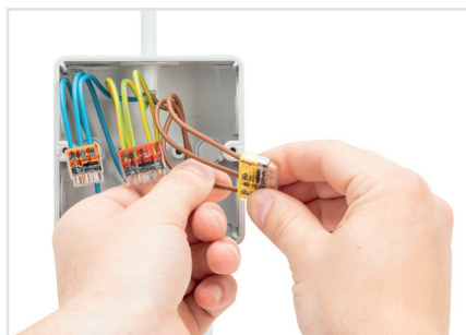
Borttagande: Håll EK ledaren som ska tas bort och vrid den fram och tillbaka samtidigt som du drar ut ledaren. FK ledare: Klipp av kabeln nära klämmans ingång, skala om den och anslut på nytt.
