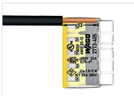
Skala EK eller FK ledaren till 13 mm
