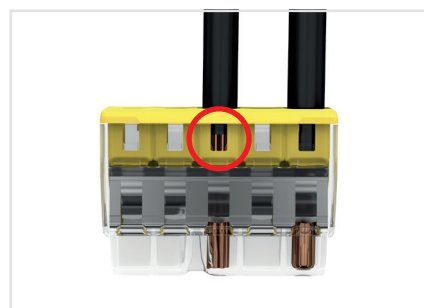
Genom det transparenta huset visas tydligt om ledaren är helt ansluten inom det färgade området, en tydlig port visar om ledarens avskalning är korrekt. Ledaren är korrekt skalad om den tydliga öppningen visar en oskalad ledare på den omärkta sidan av klämmen. Bilden visar centrerad anslutning med längre skallängd
