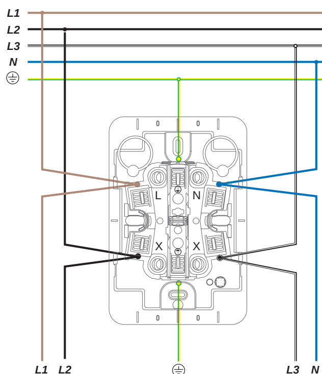
Uttag med 2 st neutrala överkopplingsklämmor
