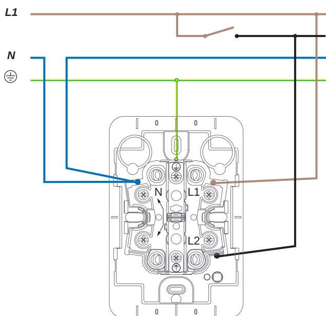
Uttag med separat brunntändning (en fas)
