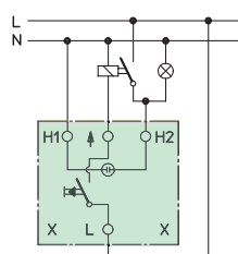
Viptryckknapp med separat lampkrets
