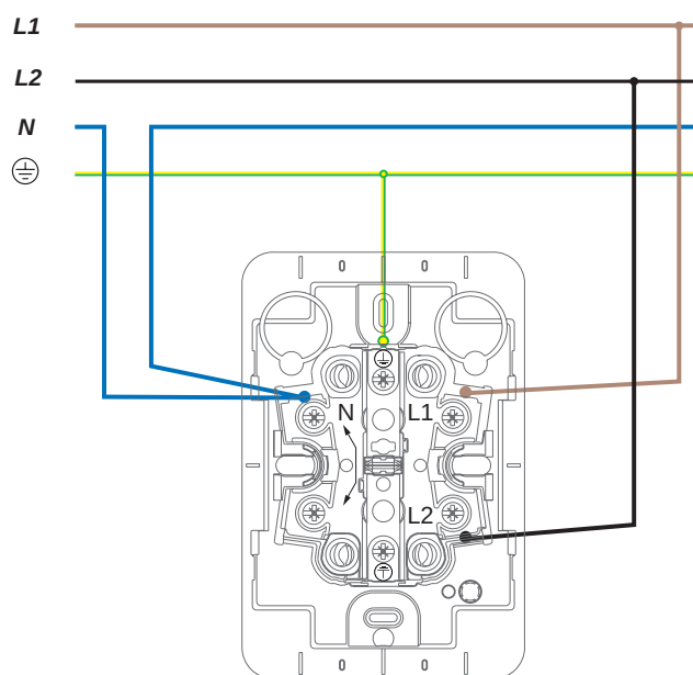
Uttag med två separata faser (440V)
