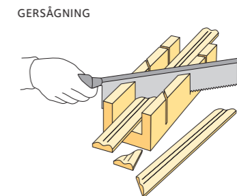
GERSÅGNING
